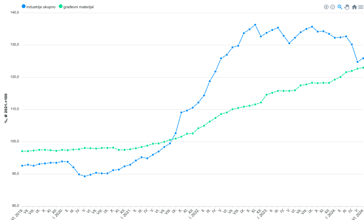
G-1. INDEKSI PROIZVOĐAČKIH CIJENA GRAĐEVNOG MATERIJALA NA DOMAĆEM TRŽIŠTU OD LIPNJA 2019. DO LIPNJA 2024. 1)
